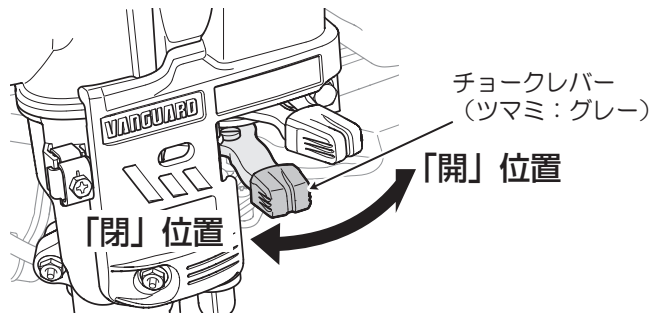
ブリグス&ストラットン (12V3)
