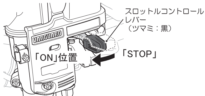
ブリッグス&ストラットン (12V3)
