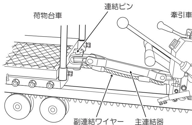
牽引車～荷物台車
