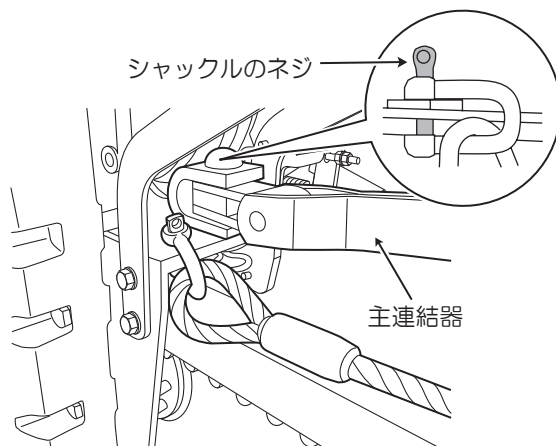
牽引車～荷物台車
